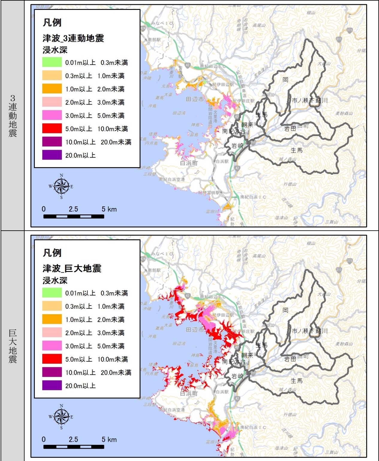
＜南海トラフの地震：津波の予測＞
