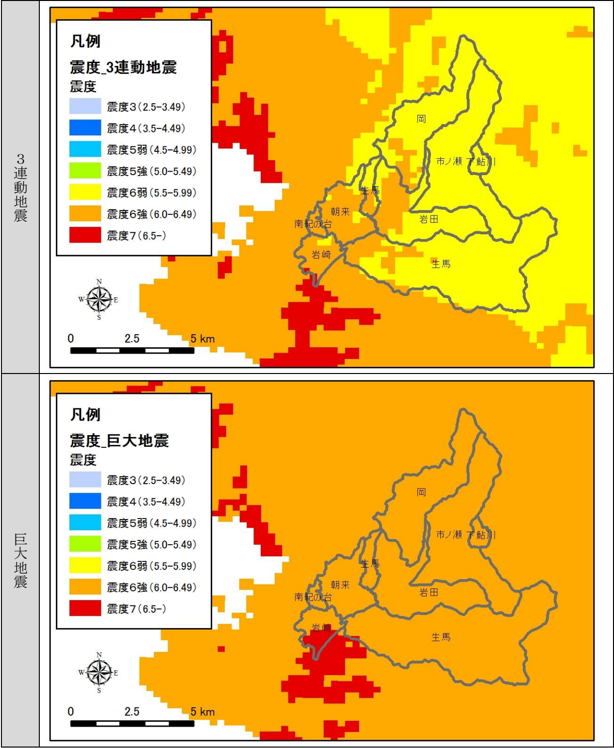
＜南海トラフの地震：震度の予測＞
